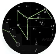
ഡിസംബർ മാസത്തെ ആകാശം
